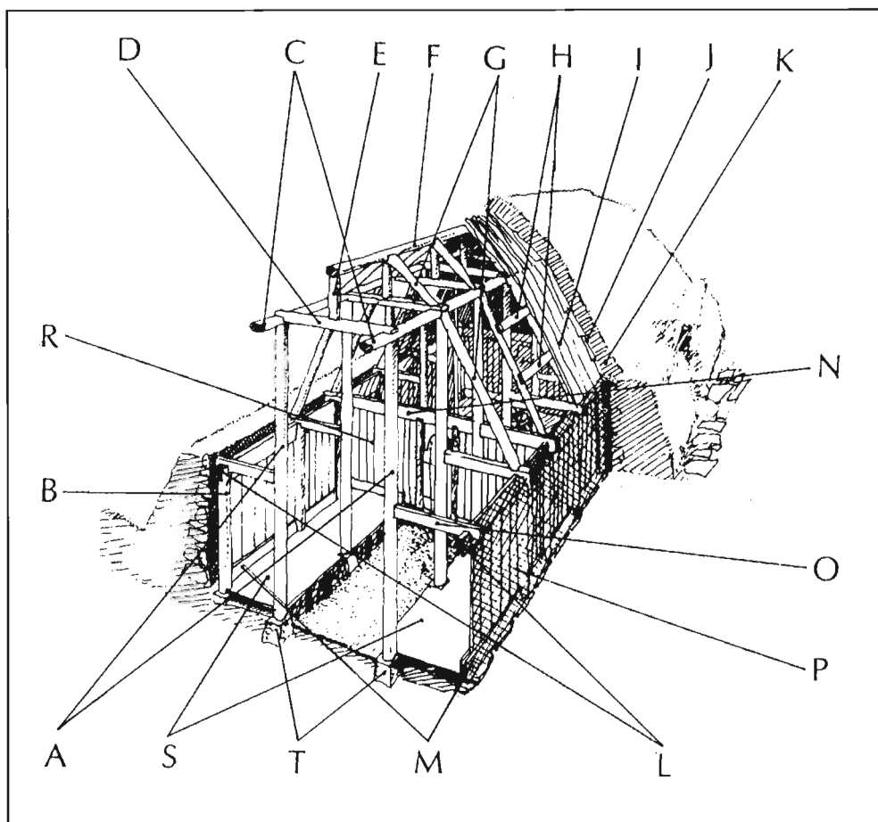
Teikning (hugmynd) Harðar Ágústssonar af skálanum á Stöng í Þjórsárdal, sem eyddist í Heklugosi 1104 og grafinn var upp 1939. Tóttin var höfð til hliðsjónar þegar „Þjóðveldisbærinn“ var byggður nálægt Skeljastöðum í sama dal 1974-77 og stóð Hörður fyrir því verki. Hér er gert ráð fyrir að skálinn sé umluktur torfgrjótveggjum og með torfþaki, en ekki er víst að svo hafi verið í upphafi hvað Valþjófsstaðaskálann varðar. (Úr þætti Gunnars Karlssonar í Sögu Íslands, II. bindi. Rvík. 1975).
